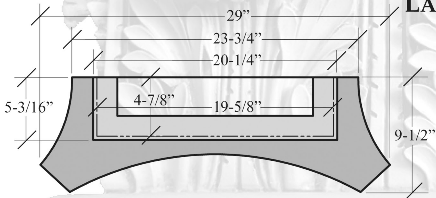
PROFILE SCALE: 1/8" = 1"
